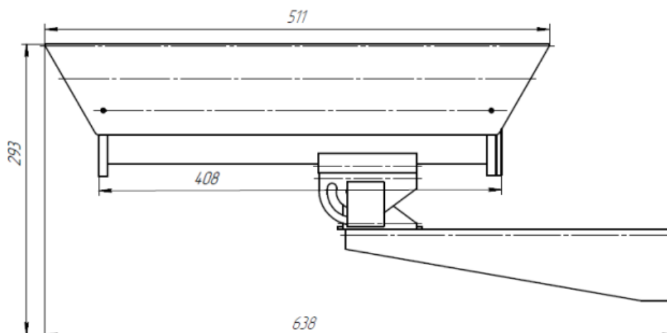
Рисунок 4.2 – Габаритные размеры термокожуха (мм)
